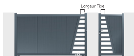
Portail Coulissant Swing Gate / Doppeltor CL31
