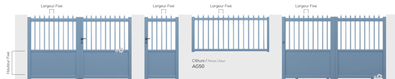
Portail Battant / Swing Gate / Doppeltor TR03B
